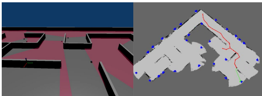
Figure 1. Le simulateur MORSE 3D (gauche) et la carte générée (droite). À gauche, la zone rouge représente le scan laser. À droite, les blocs bleus représentent les destinations potentielles, le bloc vert indique la destination actuelle, la ligne rouge le trajet déjà effectué, et la ligne verte la trajectoire pour atteindre la destination actuelle
