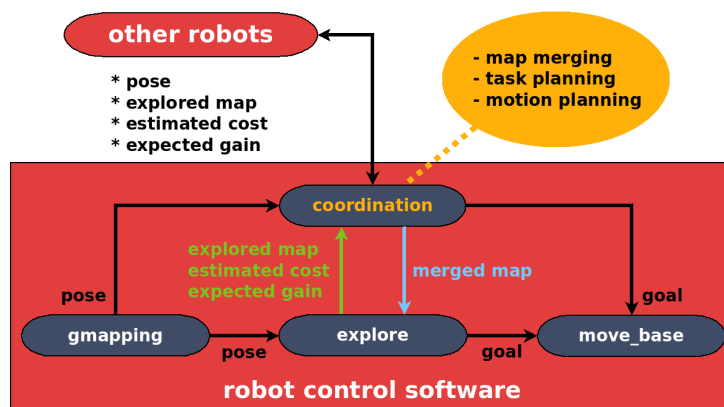
Figure 5. Architecture du logiciel de contrôle de robot
