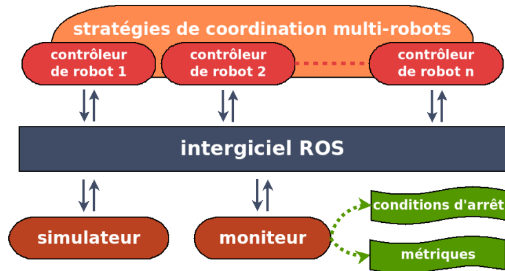
Figure 3. L'architecture du banc d'essai
