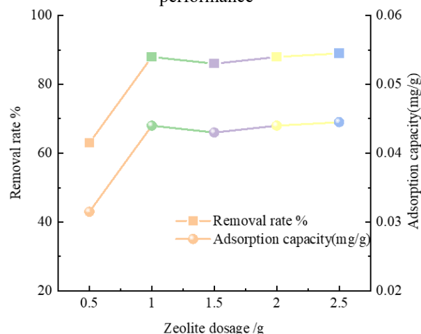
(d) Effect of zeolite dosage on adsorption performance
