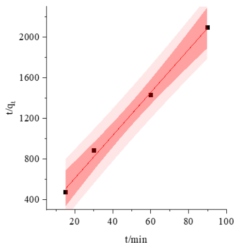
(d) Pseudo-second-order kinetics fitting trend line
